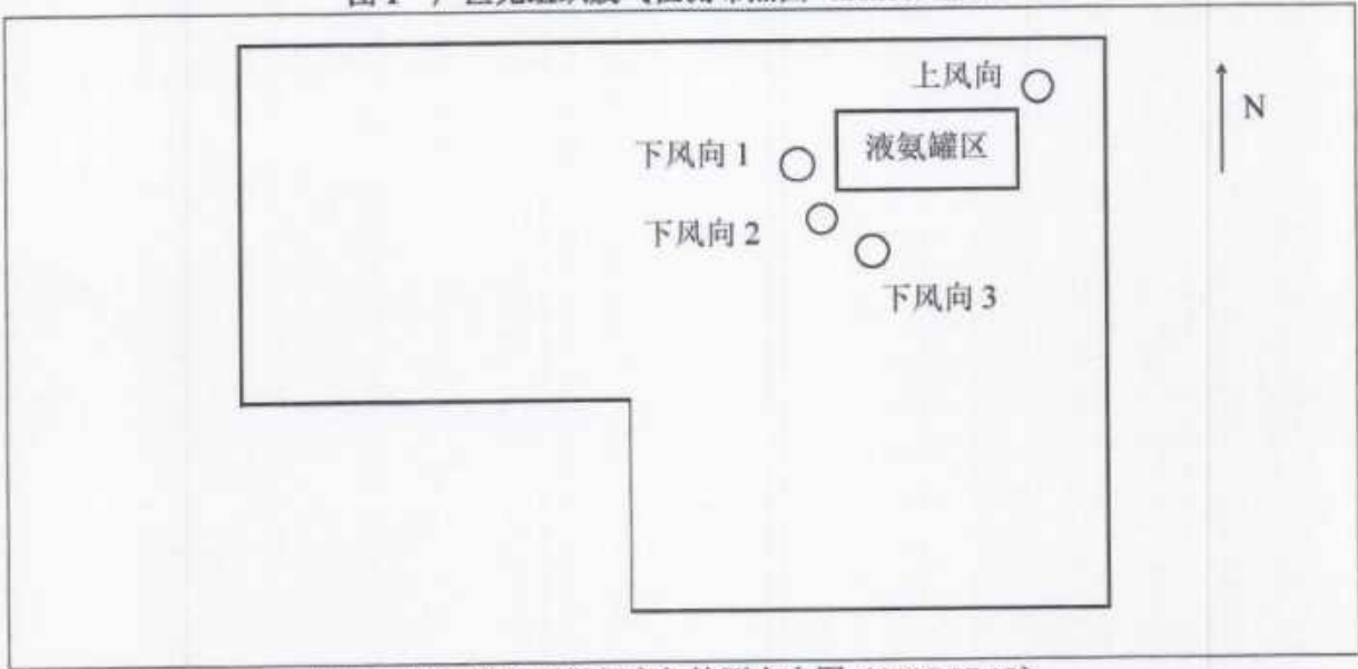
图 2 液氨罐区无组织废气检测布点图（2025.07.18）
