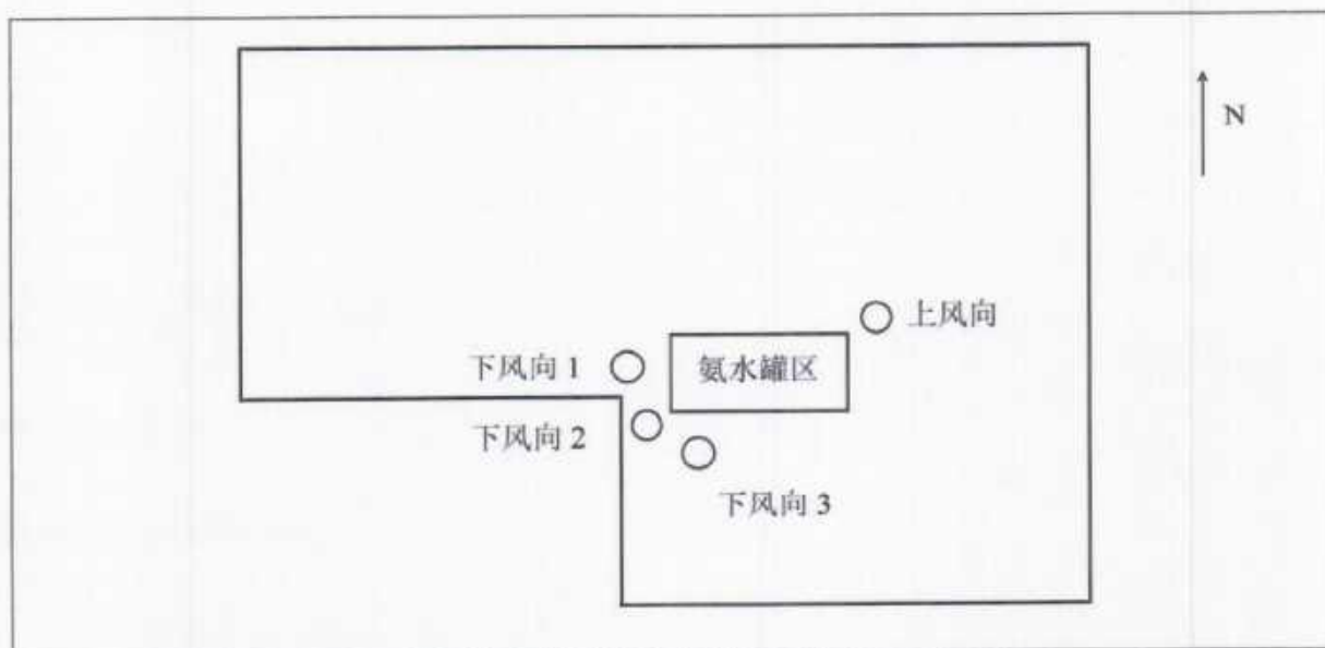
图 3 氨水罐区无组织废气检测布点图（2025.07.18）
